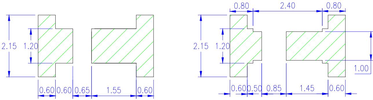
焊盘图
