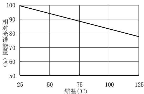
■ 结温——相对光谱能量特性曲线图
