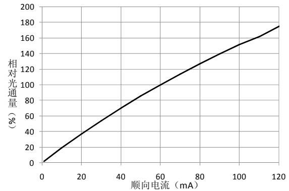
■ 顺向电流——相对光通量曲线图
