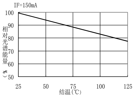
■ 结温——相对光谱能量特性曲线图
