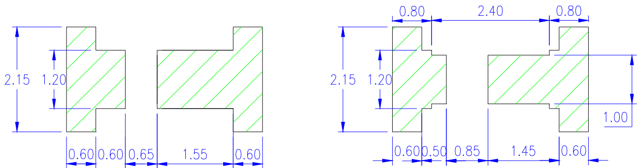
焊盘图
