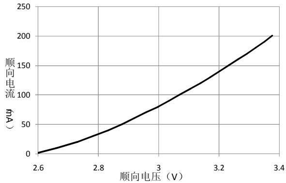
■ 顺向电压——顺向电流曲线图
