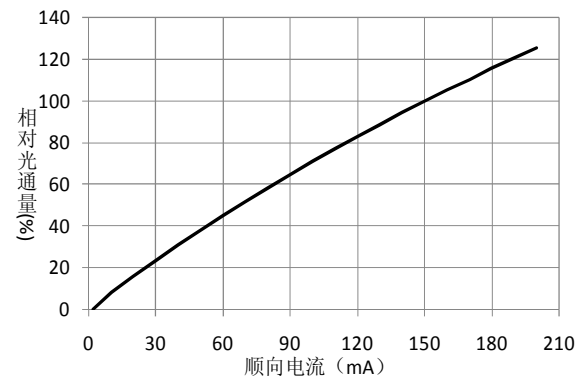
■ 顺向电流——相对光通量曲线图
