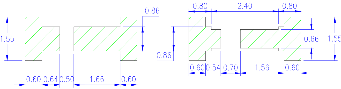
焊盘图
