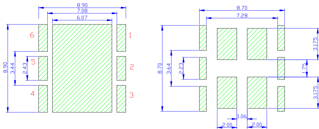
焊盘图
