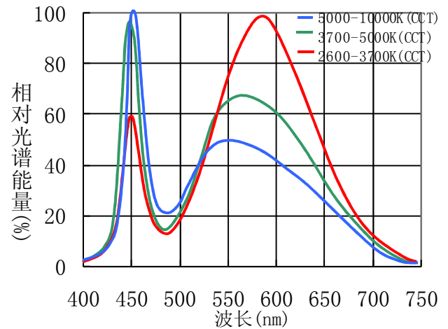
■ 相对光谱能量曲线图
