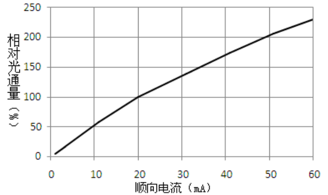
■ 顺向电流——相对光通量曲线图
