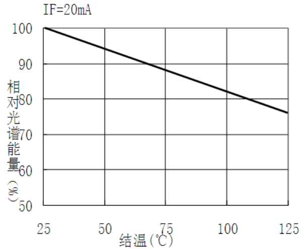
■ 结温——相对光谱能量特性曲线图
