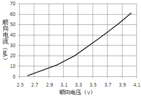
■ 顺向电压——顺向电流曲线图
