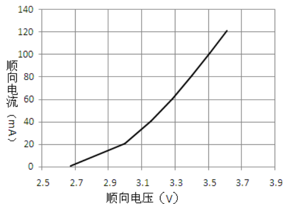
■ 顺向电压---顺向电流曲线图
