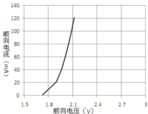
■ 顺向电压---顺向电流曲线图
