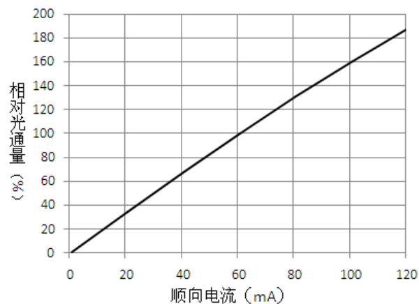
■ 顺向电流---相对光通量曲线图
