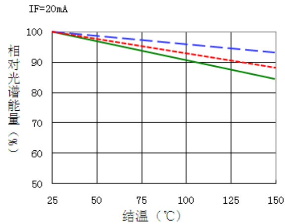
■ 结温——相对光谱能量特性曲线图
