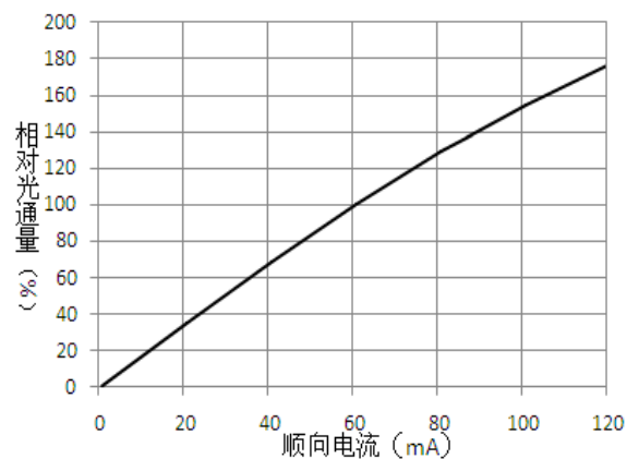
■ 顺向电流---相对光通量曲线图
