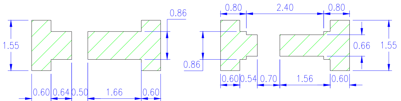
焊盘图
