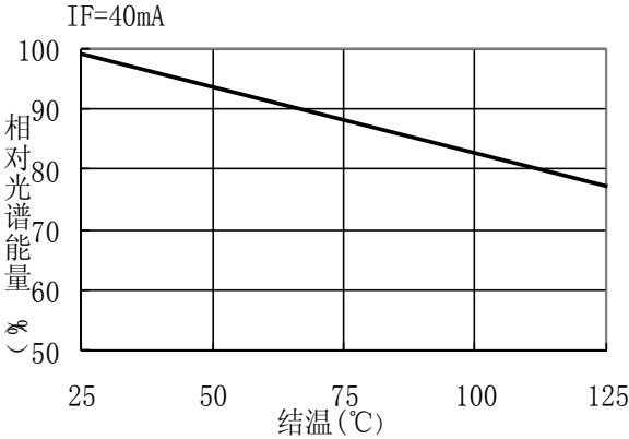
■ 结温——相对光谱能量特性曲线图
