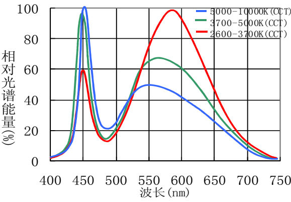
■ 相对光谱能量曲线图
