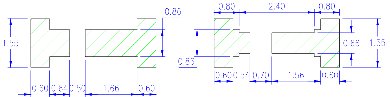
焊盘图
