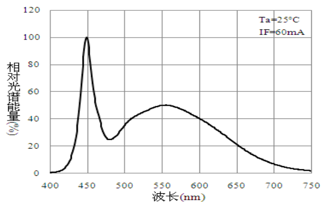
■ 相对光谱能量曲线图
