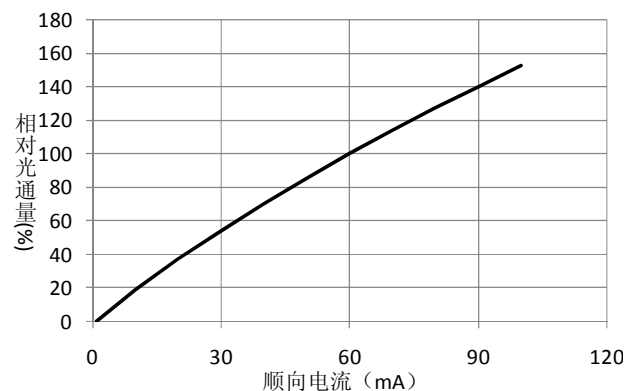
■ 顺向电流---相对光通量曲线图
