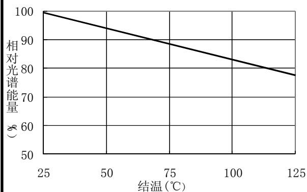
■ 结温---相对光谱能量特性曲线图
